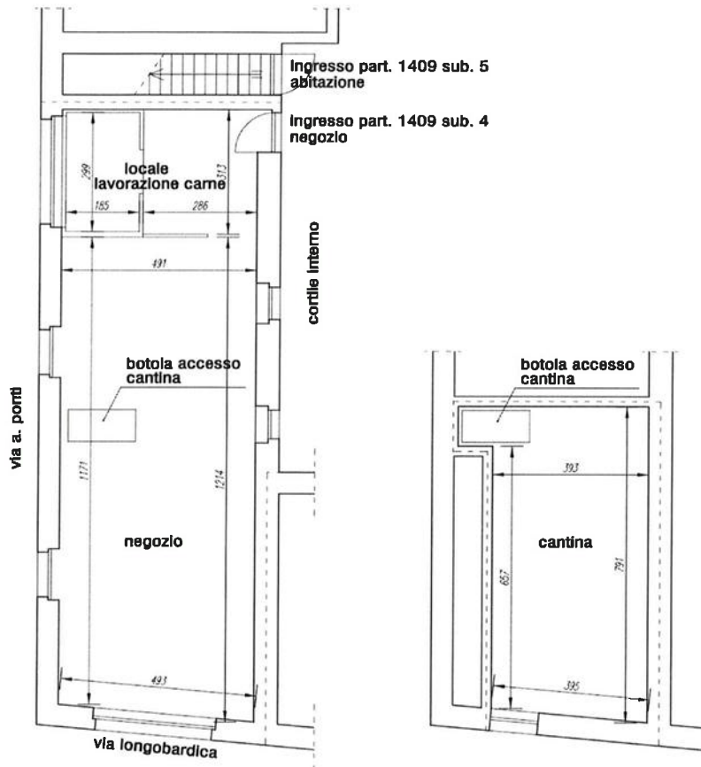
PIANO TERRA H. 305 NEGOZIO - PARTICELLA 1409 SUB. 4
