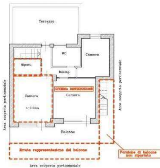
PIANTA PIANO PRIMO DA RELIEVO
