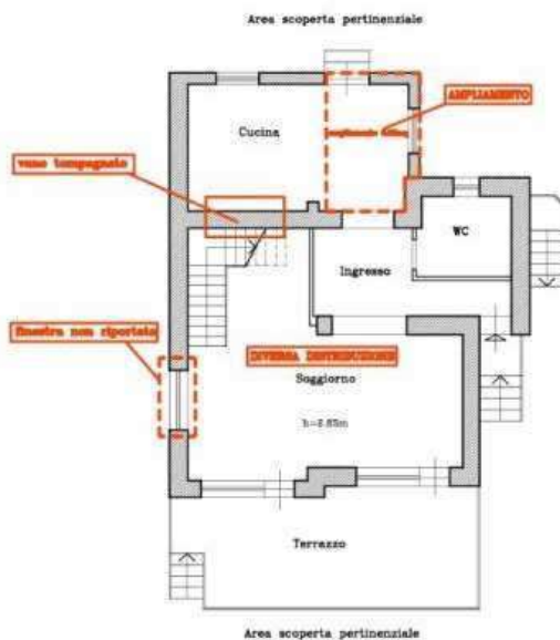
PIANTA PIANO TERRA DA RILIEVO
