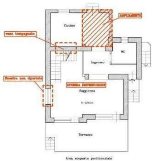
PIANTA PIANO TERRA DA RELIEVO
