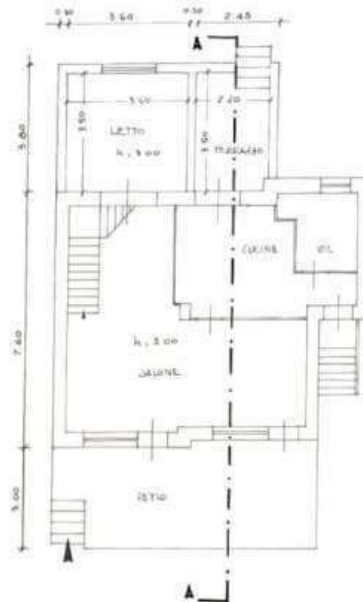
PIANTA PIANO TERRA DA CONCESSIONE EDILIZIA 902/04 DEL 07.01.2005
