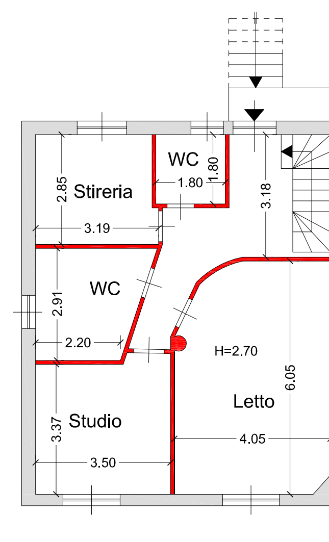
Piano Primo
