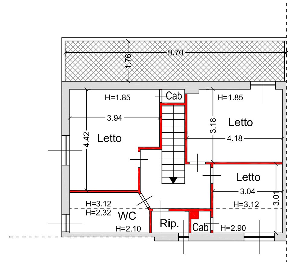
Piano Primo Sottotetto
