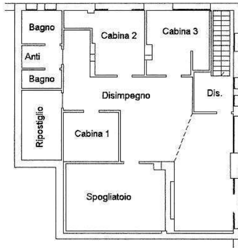
Piano Terra H= 3,00 mt.
