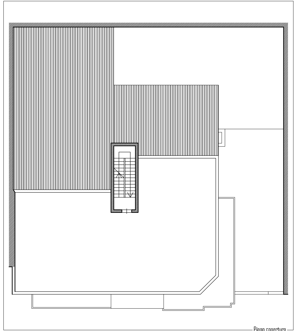
Piano copertura
