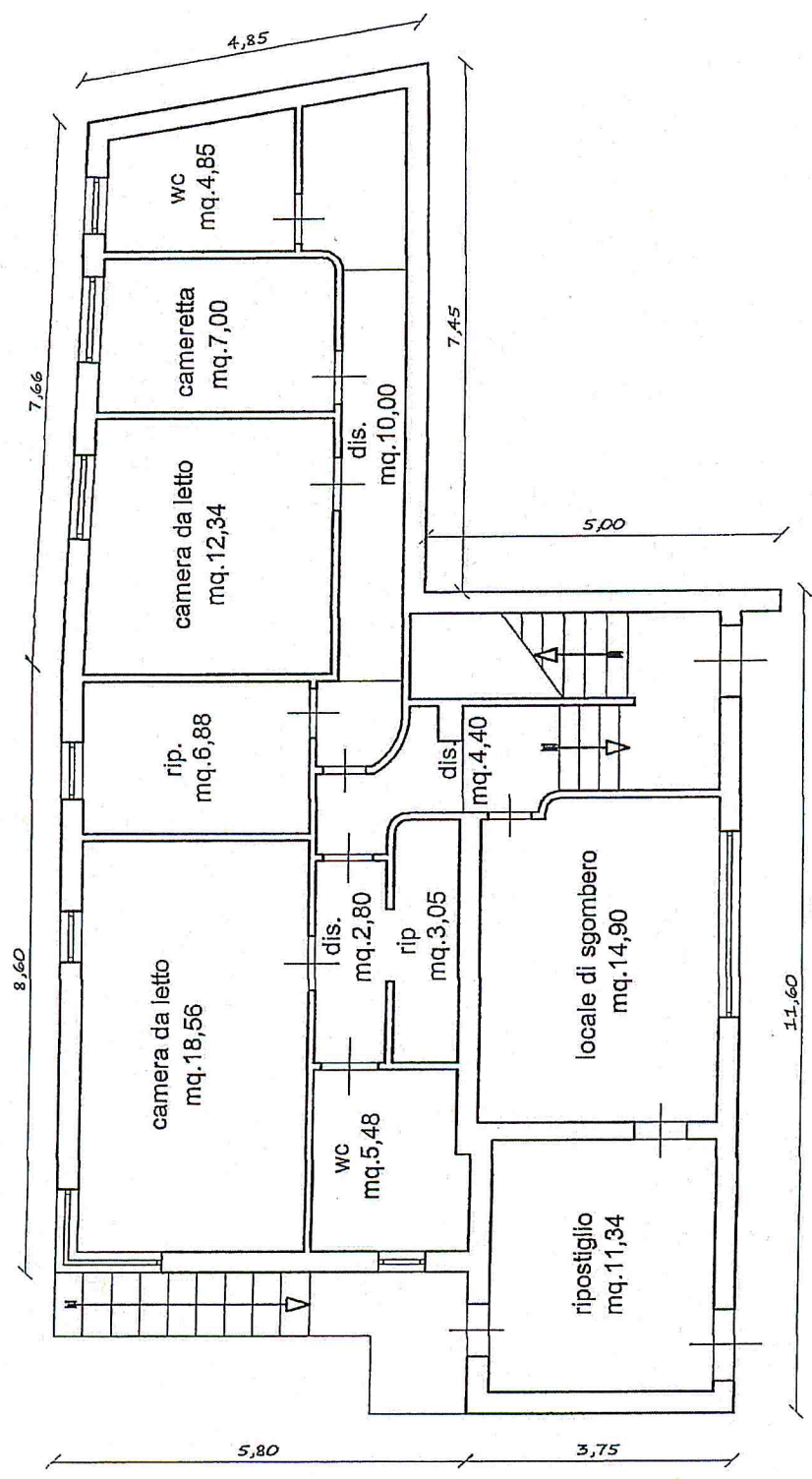
via Eleuterio pianta piano seminterrato
