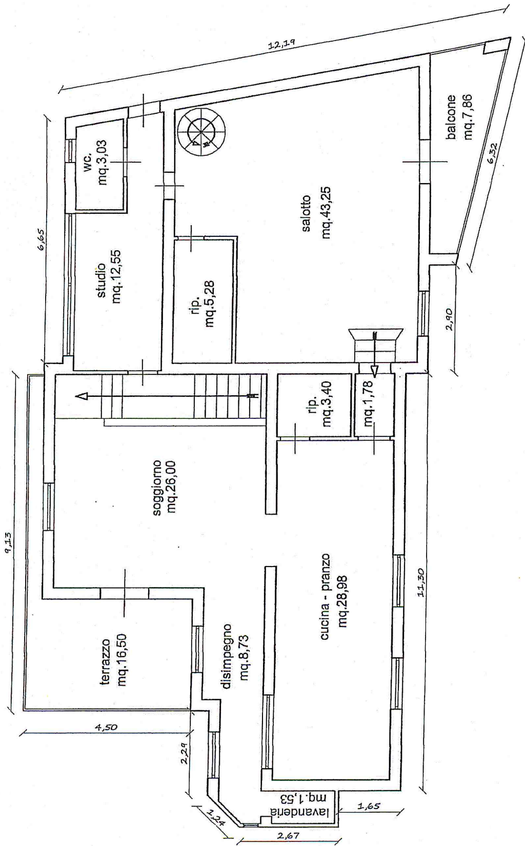
pianta piano rialzato
